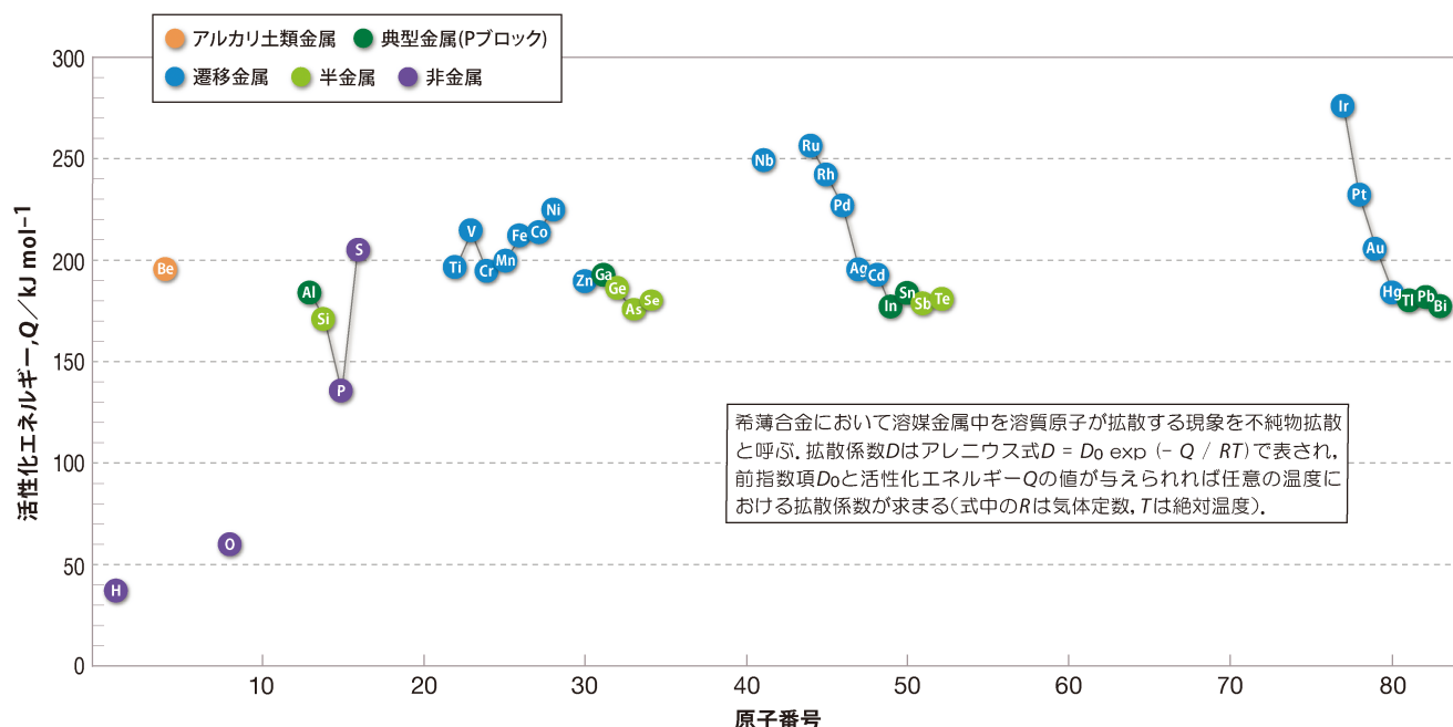
図1 銅における溶質元素の不純物拡散係数の活性化エネルギー。
