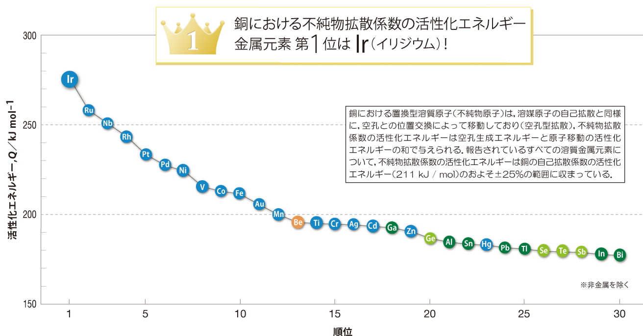
図2 銅における溶質金属元素の不純物拡散係数の活性化エネルギーランキング(上位30位まで)。
