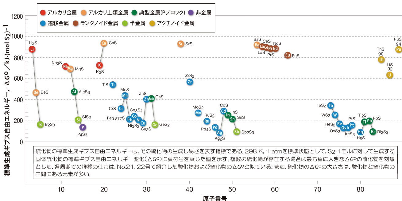
図1 各元素の硫化物に対する標準生成ギブス自由エネルギー (1)-(3) 。
