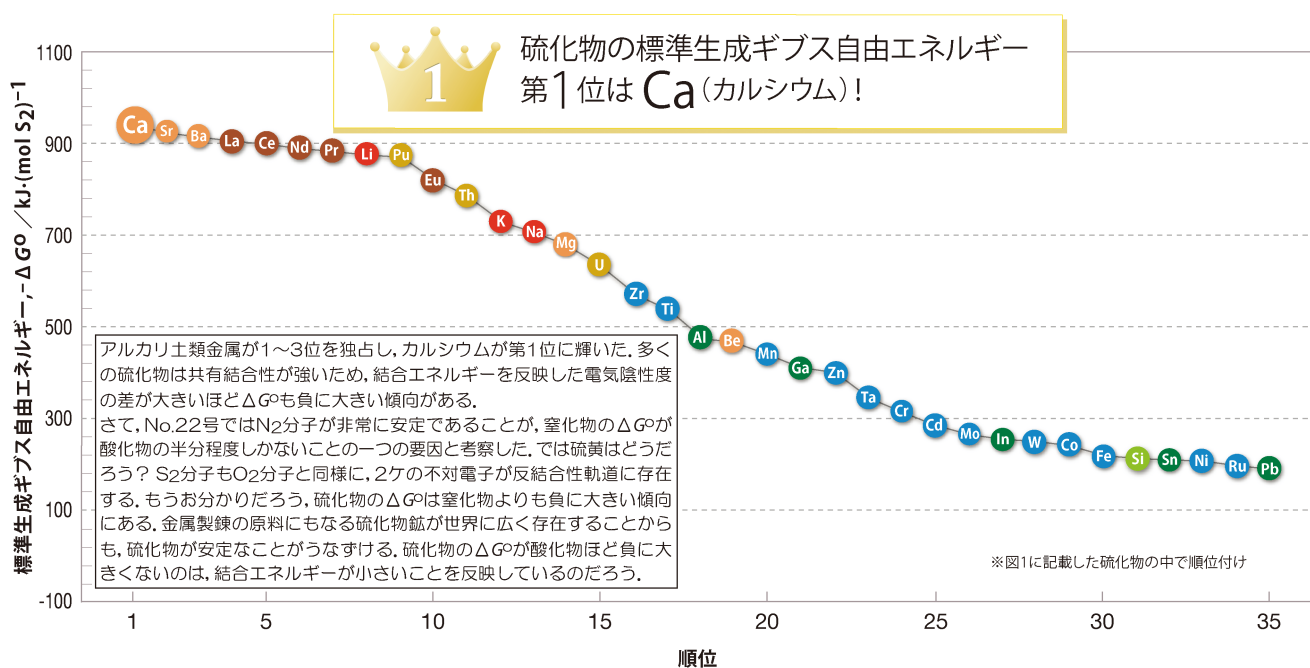
図2 硫化物の標準生成ギブス自由エネルギーに対するランキング(上位35位まで)。
